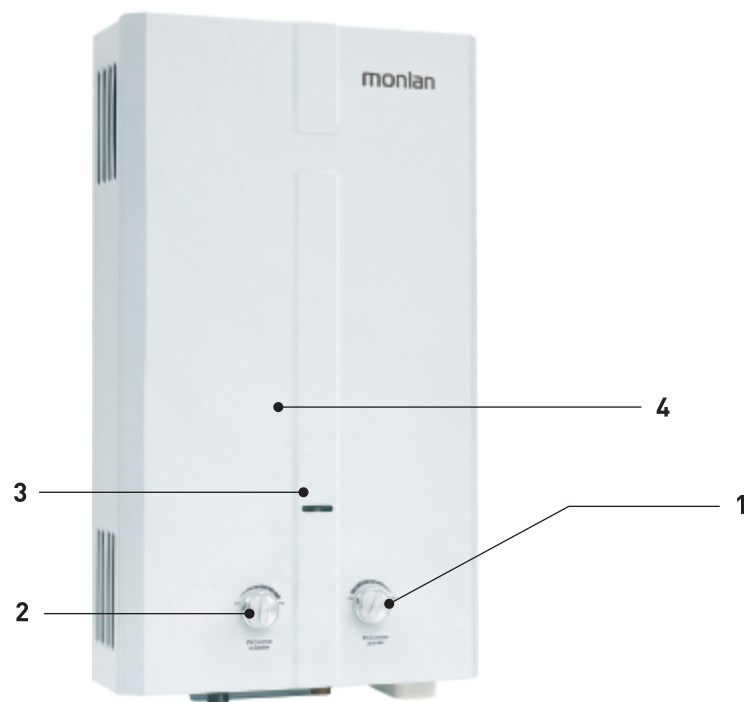
Рис. 1. Аппарат водонагревательный проточный газовый бытовой «MONLAN» 1 - ручка водяного регулятора; 2 - ручка газового регулятора; 3 - смотровое окно; 4 - облицовка.
