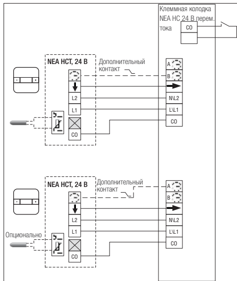
Рис. 15.8-8. Схема электрического подключения терморегуляторов NEA HCT к клеммной колодке HC 24 В
