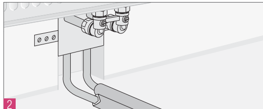
Рис. 14.4-4 Подключение отопительного прибора трубой RAUTITAN stabil при помощи присоединительного блока REHAU
