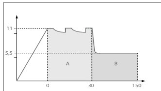
Рис. 17.2-8 Диаграмма гидравлического испытания для труб RAUTITAN flex, RAUTITAN his
