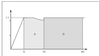
Рис. 17.2-7 Диаграмма гидравлического испытания для труб RAUTITAN stabil / RAUTITAN stabil platinum
