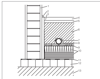
15.5-13 Шина RAUFIX с уложенной трубой RAUTHERM S в разрезе
