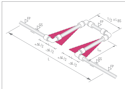
Рис. 11-2 П-образный компенсатор L_{bs} длина плеча компенсатора \Delta L температурное удлинение L длина трубы FP неподвижная опора GS скользящий хомут d_a наружный диаметр трубы, мм C константа материала трубы.
