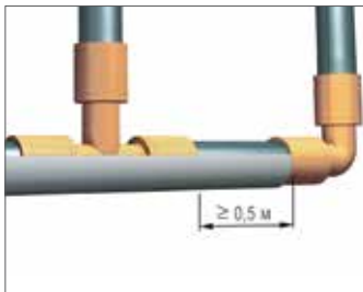
Рис. 9-4 Прокладка фиксирующего желоба поверх тройников
