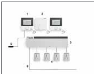
Рис. 15.9-2. Конструкция системы Nea Smart R
