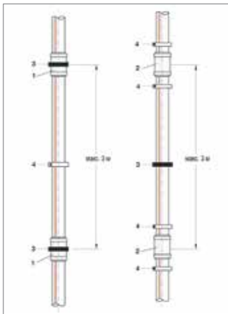
Рис. 18.1-2 Применение двухраструбных или подвижных муфт 1 Двухраструбная муфта 2 Подвижная муфта 3 Неподвижный хомут 4 Направляющий хомут
