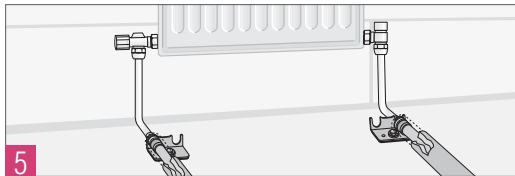
14.3-10 Подключение отопительного прибора при помощи Г-образных присоединительных трубок
