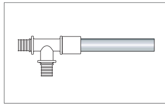
Рис 4-11 Готовое соединение
