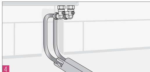
Рис. 14.4-8 Прямое подключение с помощью труб RAUTITAN stabil с отопительным прибором со встроенным вентилем
