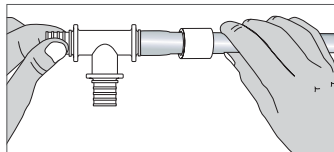
Рис 4-8 Вставка фитинга в трубу
