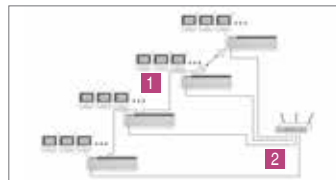
Рис. 15.9-8. Система с 4-мя клеммными колодками, объединение в сеть при помощи шин связи (1), присоединение клеммных колодок к роутеру сетевым кабелем (2)
