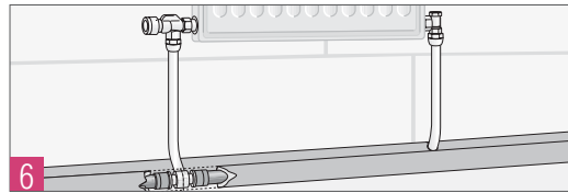
Рис. 14.3-12 Подключение отопительного прибора при помощи Т-образных присоединительных трубок RAUTITAN для разностороннего присоединения
