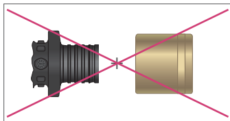
Рис. 5-1 Недопустимая комбинация фитинга RAUTITAN PX с надвижной гильзой RAUTITAN MX
