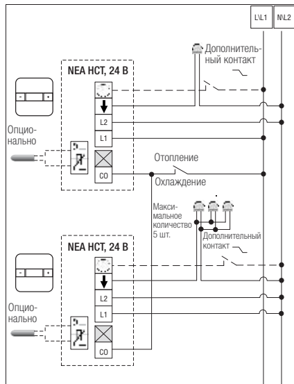
Рис. 15.8-9. Схема электрического подключения терморегуляторов NEA HCT без применения клеммной колодки NEA HC 24 В
