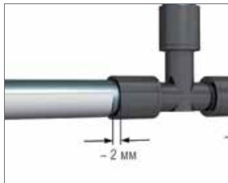
Рис. 9-5 Фиксирующий желоб недопустимо прокладывать поверх подвижных гильз RAUTITAN PX
