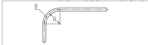
Рис. 8-2 Изгиб трубы RAUTITAN stabil
