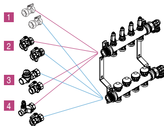
Рис. 15.7-2 Присоединительные размеры распределительного коллектора V2A НКV-D
