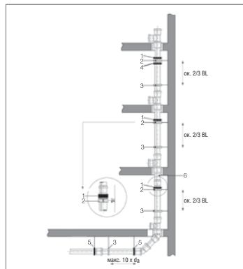
Рис. 18.2-5 Схема установки стояка
