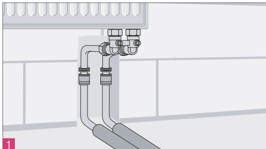
Рис. 14.4-2 Подключение отопительного прибора при помощи Г-образных соединительных трубок RAUTITAN из нержавеющей стали
