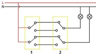
Схема цепи / Wiring Diagram
