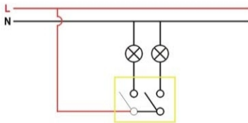
Схема цепи / Wiring Diagram
