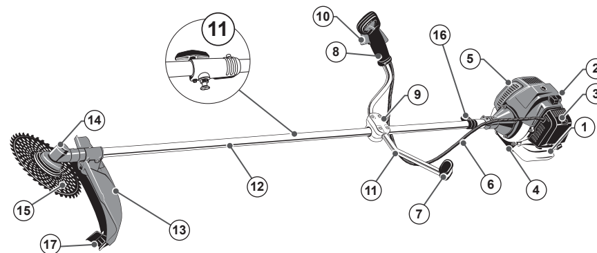
Рис.3. Расположение основных элементов бензотриммера
