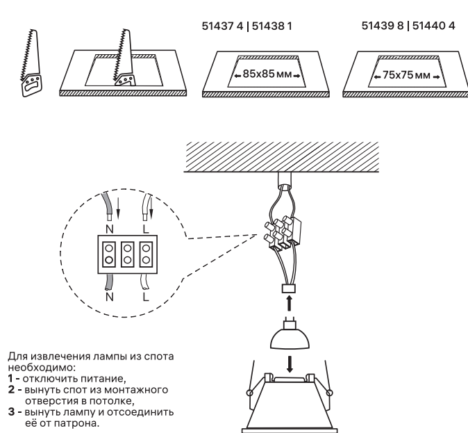
2. Монтажный комплект
