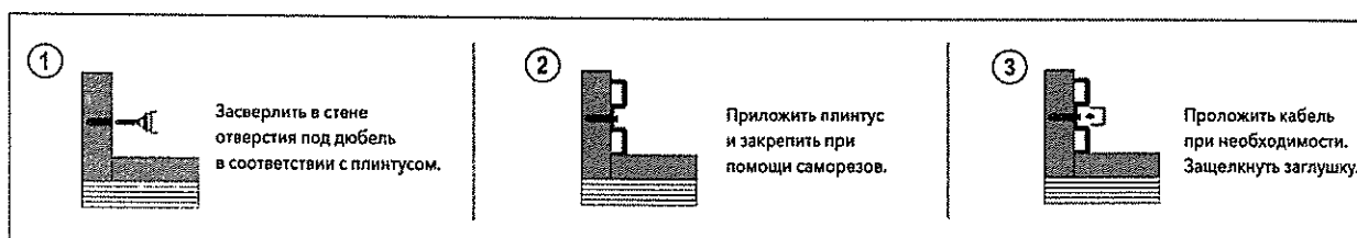
Схема монтажа 2:
